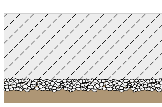
Terrændæk
