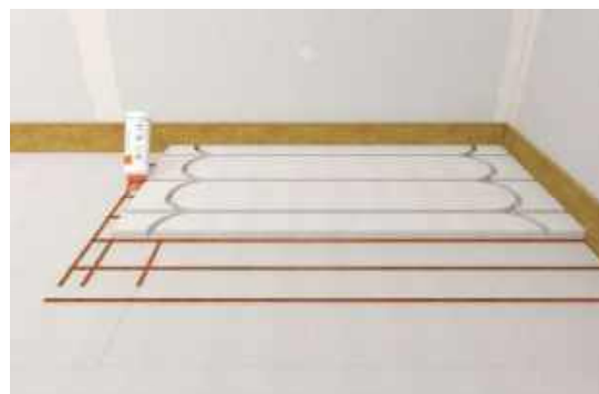
Ekstra gulvelementlim ved samlinger af Therm25™.
