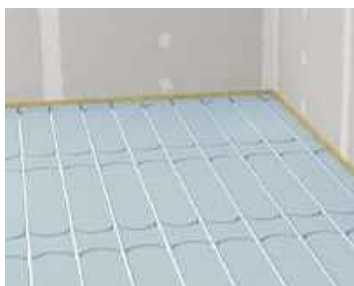
Montage af 16 mm gulvvarmeslanger
