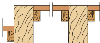
Træbjælkelag med indskud
