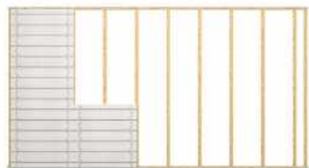
Montage af Therm25™ gulvvarmeelementer i underkonstruktionen (skruer 40 mm eller klammer 50 mm).
