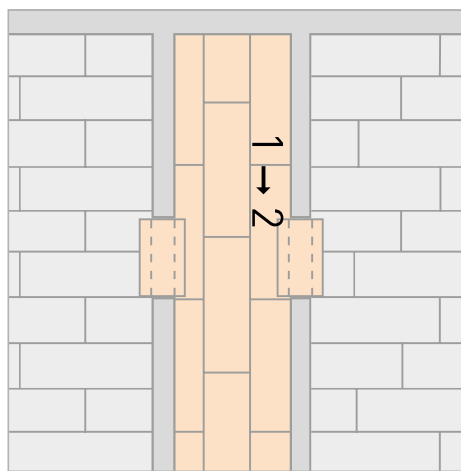
Montageskema gangarealer
