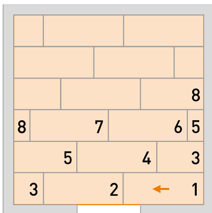
Montageskema 2
