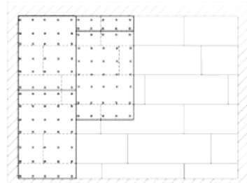
Montageskema 3. lag
