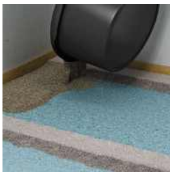
5 Vent, indtil dæmningerne er tørret. (ca. 20 minutter) Herefter udfyldes med Niveaumørtel T.
